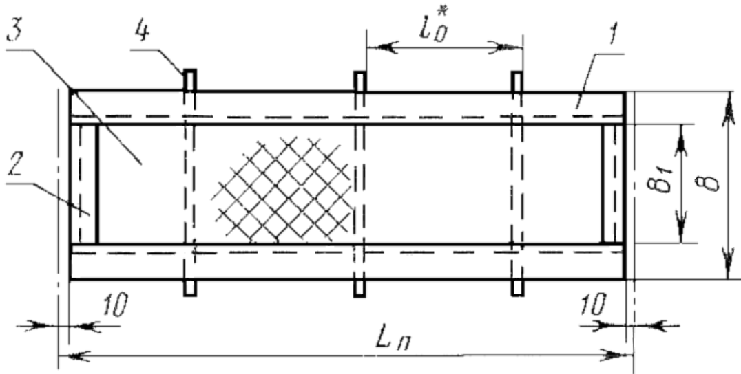
1 - балка; 2 - окантовочный элемент; 3 - настил; 4 - ребро
