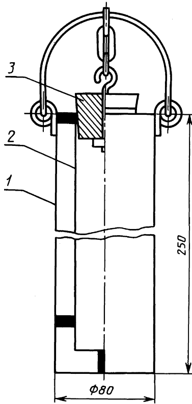
Термостатический пробоотборник
