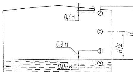
1, 2, 3, 4 - точки измерения температуры; 1, 2, 3 - точки отбора проб паровоздушной смеси
