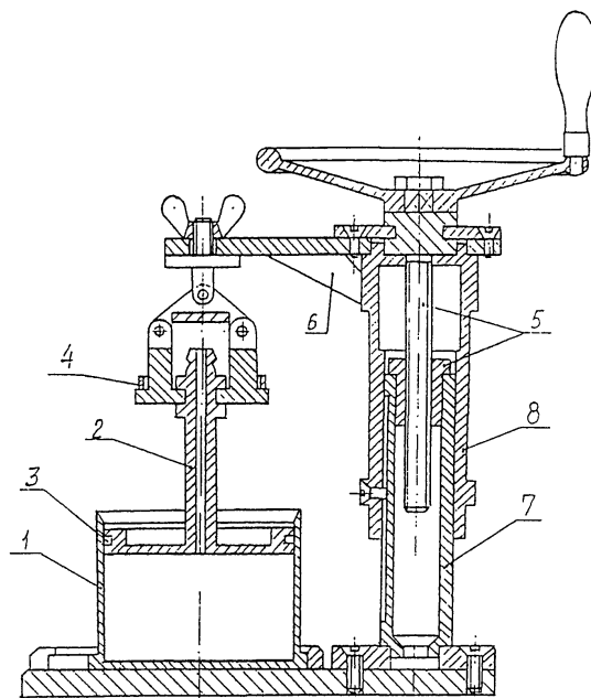
1 - стаканчик, 2 - поршень, 3 - кольцо уплотнительное резиновое, 4 - кольцо разрезное стопорное, 5 - винтовая пара, 6 - упор, 7 - направляющая, 8 - кронштейн
