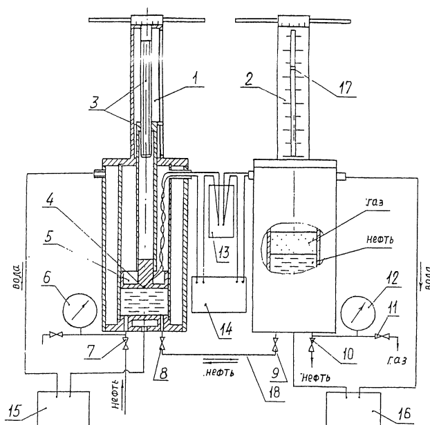
1 - аппарат первый, 2 - аппарат второй, 3 - винтовая пара, 4 - термоду, 5 - поршень, 6 - манометр, 7 - вентиль, 8 - вентиль выходной, 9 - вентиль входной, 10 - вентиль выходной, 11 - вентиль для отбора газа, 12 - манометр, 13 - сосуда Дюара для льда, 14 - потенциометр ПП-63, 15 - термостат, 16 - термостат, 17 - указатель, 18 - трубка
